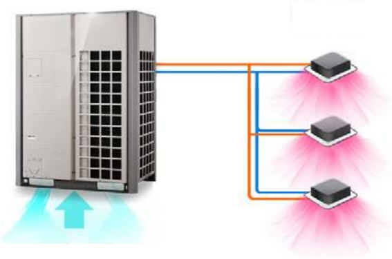
MODALITÀ RISCALDAMENTO
